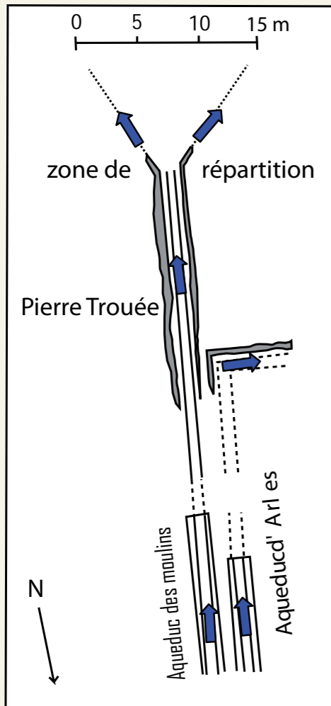
Arrivée de l'aqueduc des moulins et départ de l'aqueduc d'Arles (L. Marlin, d'après F. Benoit, Revue archéologique, 1940, 1)
