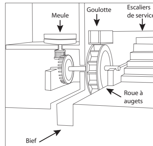
Reconstitution du mécanisme du moulin de Barbegal (L. Martin, d'après J.-P. Adam)
